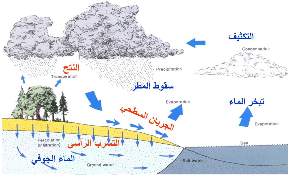
شكل يوضح دورة الماء في الطبيعة والعمليات المصاحبة لها
